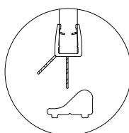
Détail C
