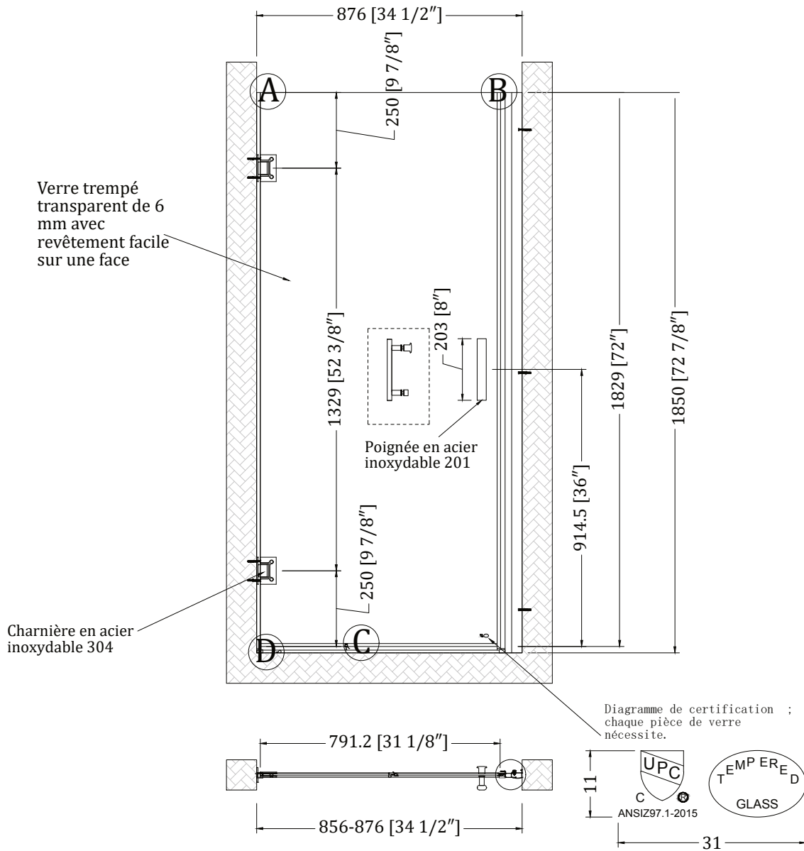
Dimensions d'un mur à l'autre (856mm-876mm)
